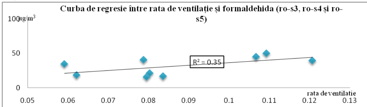
Graficul 4.4.9 Curba de regresie între rata de ventilație și conc.de formaldehidă din ro-s3, ro-s4 și ro-s5
